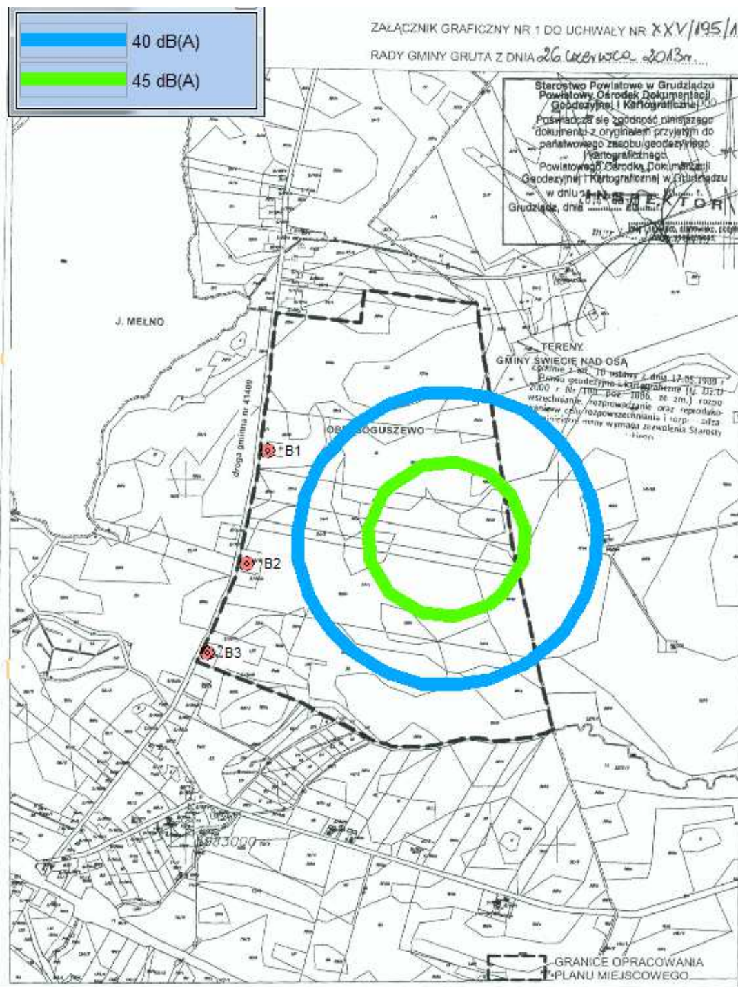
Mapa izofon obrazująca propagację hałasu dla 1 siłowni wiatrowej
