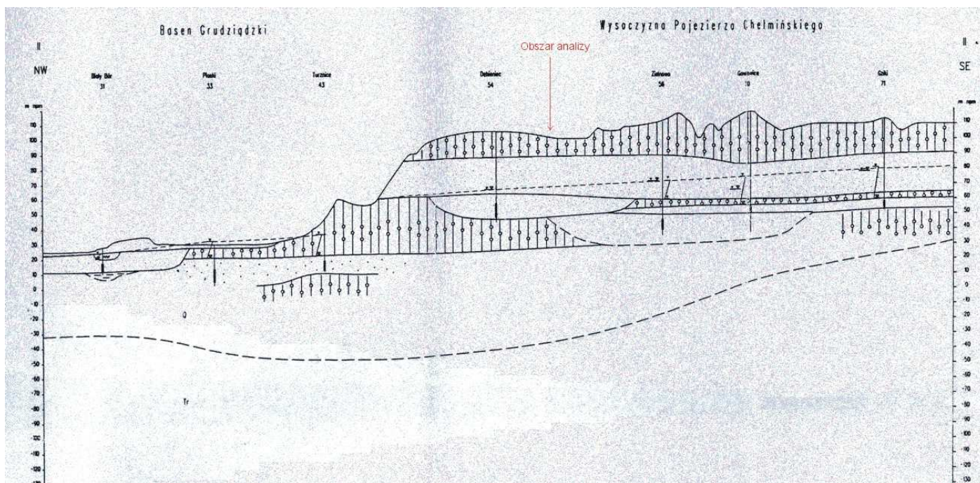
Przekrój geologiczny
