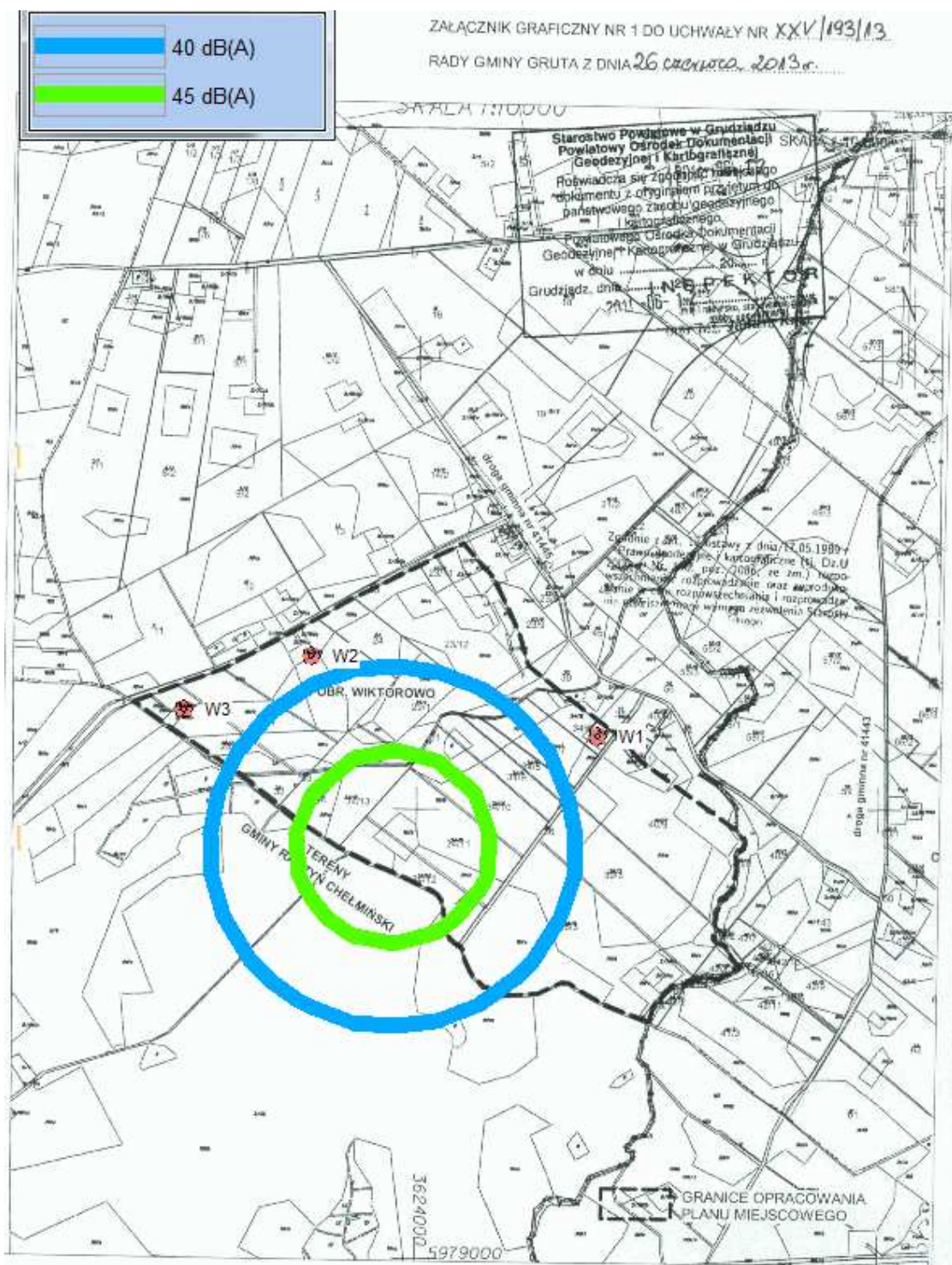
Mapa izofon obrazująca propagację hałasu dla 1 siłowni wiatrowej
