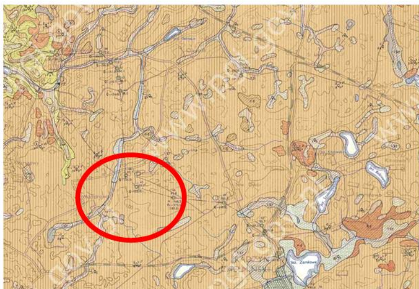
Rys. nr 4. Wycinek ze szczegółowej mapy geologicznej Polski z zaznaczonym orientacyjnie położeniem obszaru objętego mpzp.
