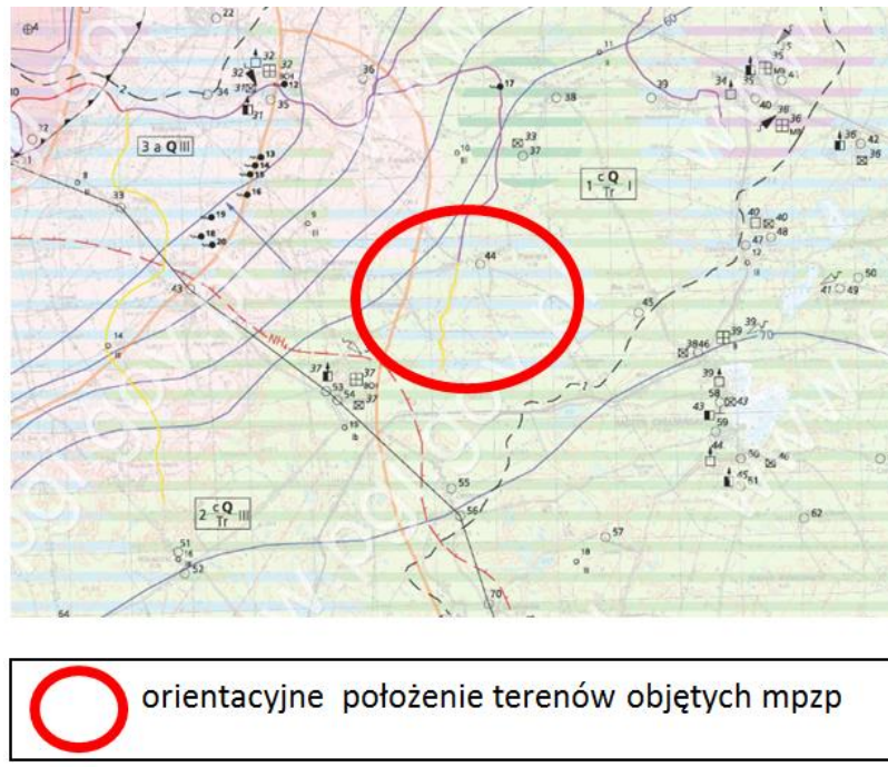
Rys. nr 5. Wycinek z mapy hydrogeologicznej z orientacyjnie zaznaczonym terenem opracowania.
