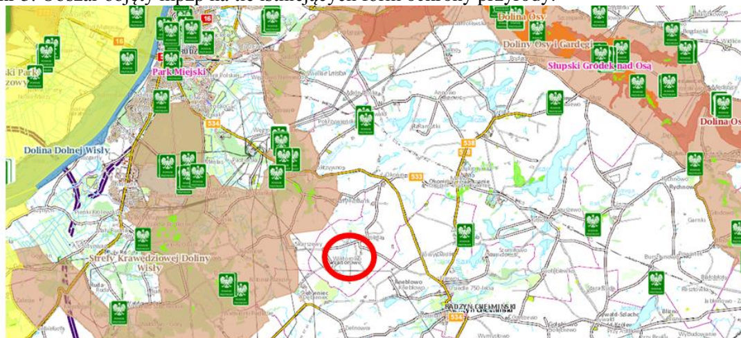
Rys. nr 3. Obszar objęty mpzp na tle istniejących form ochrony przyrody.
